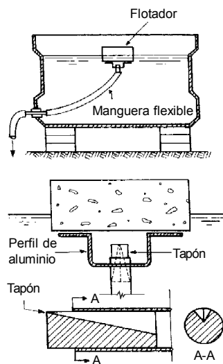
Figura 6-16. Hipoclorador de orificio de carga constante (4)
