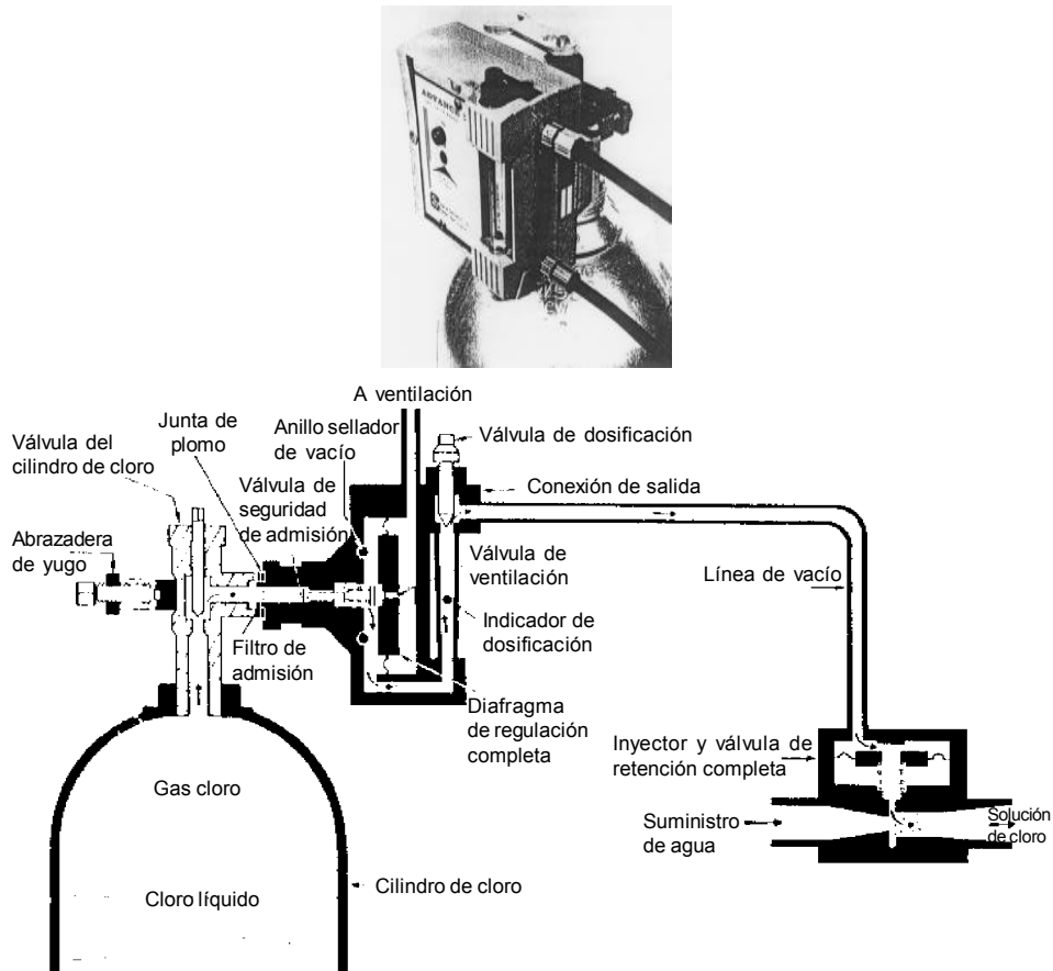
Figura 6-25. Diagrama de flujo de un clorador de aplicación al vacío (3)
